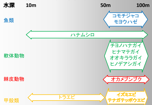
共通分類群
