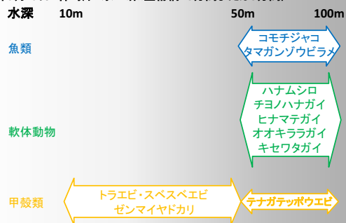
共通分類群
