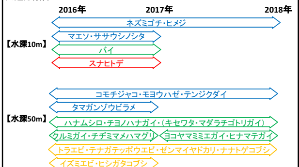
共通分類群
